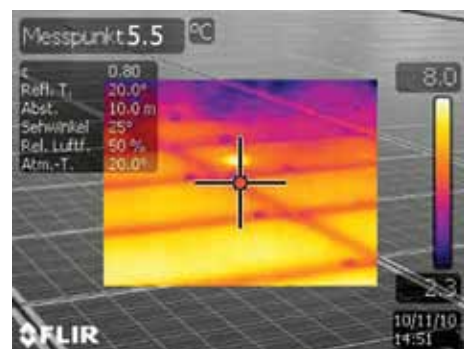
Mittels der Bild-im-Bild-Funktion kann der Bediener das Wärmebild direkt über das entsprechende Realbild legen. Er kann per Tastendruck Wärmebilder einfach innerhalb des Realbilds bewegen sowie ihre Größe und Form verändern.
