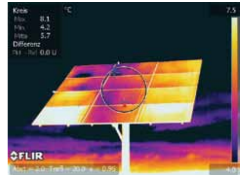
Die heißen Stellen auf diesem Wärmebild, das von der Vorderseite des Solarmoduls aufgenommen wurde, könnten ein Anzeichen dafür sein, dass eine Vielzahl von Zellen ineffizient arbeitet.
