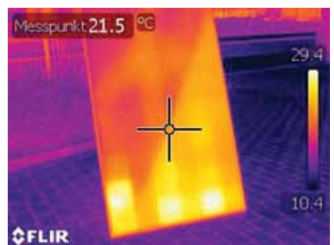
Ein Test mit einem Solarmodul auf dem Parkplatz von Solartechnik Stiens zeigt, dass die heißen Stellen sogar von vorne mühelos auf dem Wärmebild zu erkennen sind.
