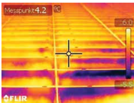
Dieses Wärmebild zeigt deutlich, dass Reflexionen bei der Inspektion von Solarmodulen ein Problem darstellen können: Die Wärmebildkamera nimmt das reflektierte Wärmebild der Wolke auf, anstatt die Temperatur des Moduls zu messen.
