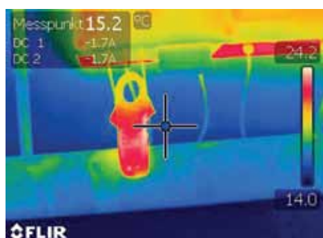
Mit der FLIR MeterLink-Technologie lassen sich die vom Zangenmessgerät erfassten Messdaten via Bluetooth übertragen und mit dem Wärmebild verknüpfen.
