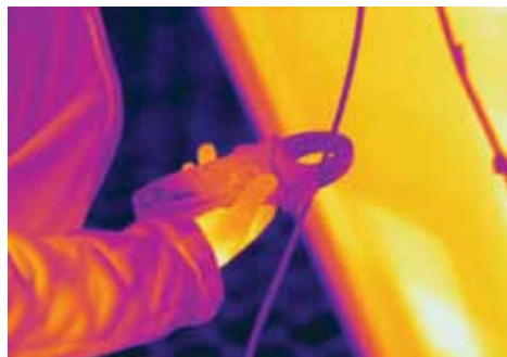
Die vom Modul produzierte Strommenge kann recht einfach mit dem Zangenmessgerät ermittelt werden. Die Messdaten werden mithilfe der FLIR MeterLink-Technologie mit dem Wärmebild verknüpft.
